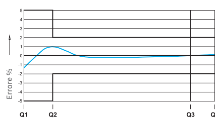
Q_1 = Portata minima Q_3 = Portata permanente Q_2 = Portata di transizione Q_4 = Portata di sovraccarico massima
