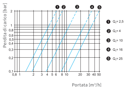
Tipica curva delle perdite di carico
