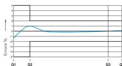
Tipica curva degli errori
