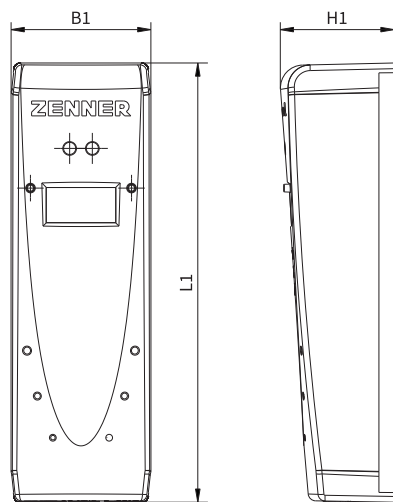
Abmessungen Kompaktversion
