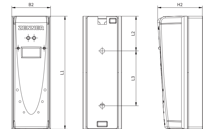
Abmessungen Splittversion
