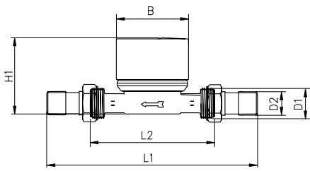
Méretek
