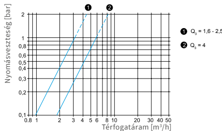
Tipikus nyomásvesztési görbe
