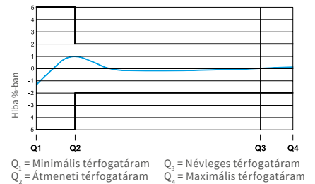
Tipikus hibagörbe
