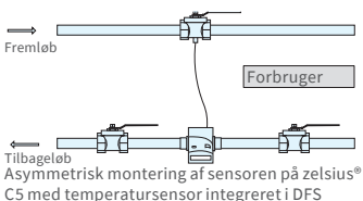
Monteringseksempel for messingforskrning
